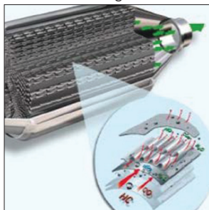
Onderhoudsvrij roetfilter
